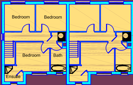
Type F1 First Floor Plan
